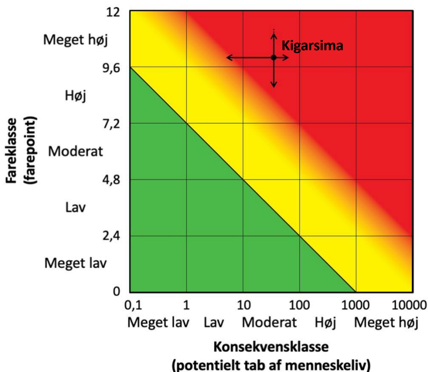
Ilusiliaq 12: Kigarsimamut aarlerinaataasunut ilusiliineq. Navianartoqarnerata nalorninartoqarnerani takuneqarsinnaavoq navianartunut tunngavissarititaasut ilaanni paasisutissat nalunaarsukkat tunngaviusut killeqarnerat, qaqqani ilutsini nunap sannaanut tunngasut, maannakkut pisoqarnera aammalu sumiiffinni siusinnerusukkat qaqqaq sisoorluni pisoqartarsimanera takuneqarsinnaallutik. Kingunerisassat annertussilerneqarneranni nalorninartortaasuni, pivusorsioortumik sisoornernut takorluukkat assigiinngisitaarnerat, aammalu qaqqap sisoornera tininngatillugu aammalu ulissimatillugu pisinnaasoq, takuneqarsinnaapput. GEUS-ip allakkiaanit 4. oktober 2022a-meersumit.
