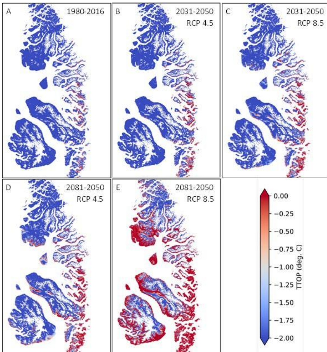
Ilusiliaq 20. Piffissami A) 1980–2016, B) 2031–2050 Kalaallit Nunaata kitaani nunap qeriuannartup qaavani nunap qaleriiaarnerini (TTOP) agguaqatigiissillugu kissassutsit pisuusaartinneqartut, RCP 4.5-imi siumut naatsorsukkat aallaavigalugit, C) 2031–2050 RCP 8.5-imi siumut naatsorsukkat aallaavigalugit, D) 2081–2100 RCP 4.5-imi siumut naatsorsukkat aallaavigalugit, E) 2081–2100 RCP 8.5-imi siumut naatsorsukkat aallaavigalugit. Malugiuk, ilusiliani nunap qaavata ataani itisuumi nunami qeriuannartumi kissassusissat pisuusaartitsivigineqanngillat. Taamaattoq TTOP pisuusaartinneqartup annertusineqarnera paasineqassaaq, piffissap ingerlanerani kissatsikkiartornerata ingerlasup kingunerisaanik itisuuni nunap qeriuannartup annikilliartornissaanik naggataatigullu qeriuannaarnissaanut tamanna tikkuussisooq. Uinganerit -2^{\circ}\text{C} – 0^{\circ}\text{C} akornanni qajannarnerusarput.
