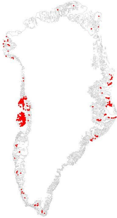
Ilusiliaq 6: Qaqqat sisoorneri Kalaallit Nunaanni kingullermik sermeqarnerata nalaata kingorna pisimasut. Toornerni aappaluttuniipput qaqqat sisoornerisa unerarfi imaluunniit qaqqap sisoornerata kingorna itersannguunnerit. Svennevig-ip ilusiliaa (2019).
