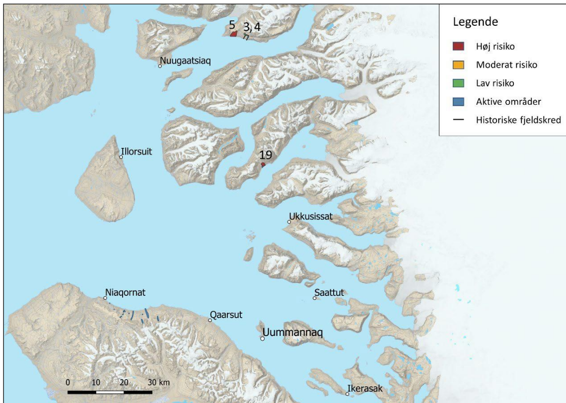
Ilusiliaq 3: Uummannaq sulluata avannarpasinnerusortaanut nunap assinga sukumiisoq InSAR-imi nikikkiartuaartunik qaqqat qajannartortallit sumiiffiillu pisoqarfiusut nalunaaqutserneqarlutik. Qaqqat nalunaaqutsigaasut tassaapput Karrat 1 (nr. 3), Karrat 2 (nr. 4), Karrat 3 (nr. 5) aamma Kigarsima (nr. 19).
