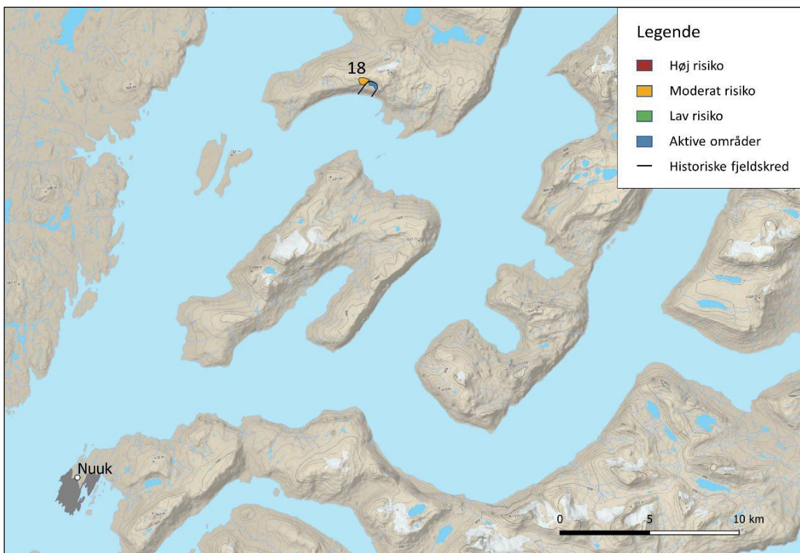
Ilusiliaq 5: Nuup Kangerluata kujasinnerusortaanut nunap assinga sukumiisoq, qaqqat qajannartortaqtartut aamma sumiiffiit pisoqarfiusut InSAR-imi nikikkiartuaartut nalunaaqutserneqarlutik. Qaqqaaq nalunaaqutserneqartoq tassaavoq Qaarusuup Qaqqaa (nr. 18).
