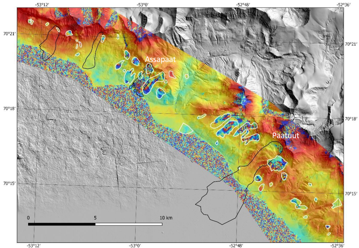
Ilusiliaq 17: Nuussuup kujammut sineriaata qiterpasinnerusortaa InSAR interferogram atorlugu tigusaq 20. – 26. juli 2021 (kujammuinnaq sammisoq 25), hillshade af ArcticDEM qaavani tigusaq. Sumiiffiit InSAR-imi nikikkiartuaartortallit qaqortumik titarnilerlugit nalunaaqutserneqarput, aammalu qangarsuaq qaqqat sisoortarsimani qernertumik titarnilerlugit nalunaaqutsigaallutik. Qangarsuaq qaqqat sisoortarsimani marluk Paatuuni 1996-imi aamma 2000-imi pisimapput. Malugiuk Assapaani 13. juni 2021 qaqqap sisoornerata sisoorfiani InSAR-imi malugineqartoq nipiliorfiusimasoq.
