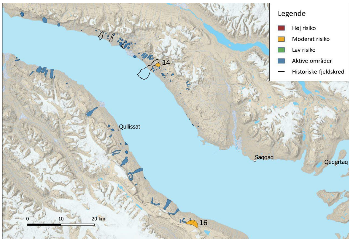
Ilusiliaq 4: Vaigat-ip ikerasaanut nunap assinga sukumiisoq, qaqqat qajannartortallit aammalu sumiiffiit pisoqarfiusut InSAR-imi nikikkiartuaartut nalunaaqutserneqarlutik. Qaqqat nalunaaqutsigaasut tassaapput Paatuut Kangia (nr. 14) aamma Illorsuaasaq (nr. 16).
