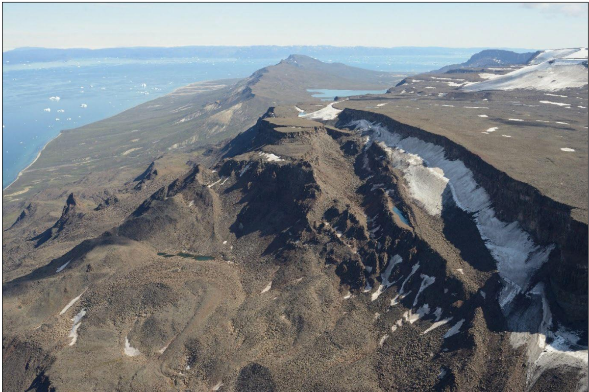
Ilusiliaq 14: Qulimiguulimmiit tukimuinnaq assilisaq, Illorsuaasami ujarasussuit qullersaanniit kangimuinnaq isigalugu. 950 meterinik portussusilimmi ujarasussuk qulleq 15 m missaannik ammuinnaq nikissimavoq aammalu quppanit sermimik ulikkaartunit toqqinnertaaniit avissaartilluinnarneqarsimasunik.
