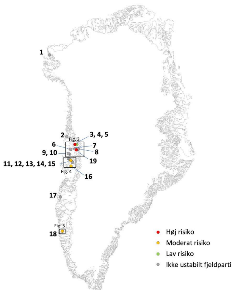
Ilusiliaq 1: "Kalaallit Nunaanni annertuumik qaqqanik sisoortoqarsinnaanera aarlerinaateqarneranik misissuinermi" sumiiffiit 19-it.
