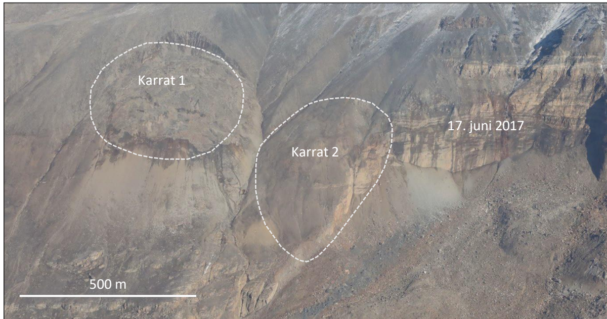
Ilusiliaq 16: Karrat 1-imut aamma 2-mut kiisalu 17. juni 2017 sisoorfusup ilaanut qulimiguulimmit tukimuinnaq assilisaq.
